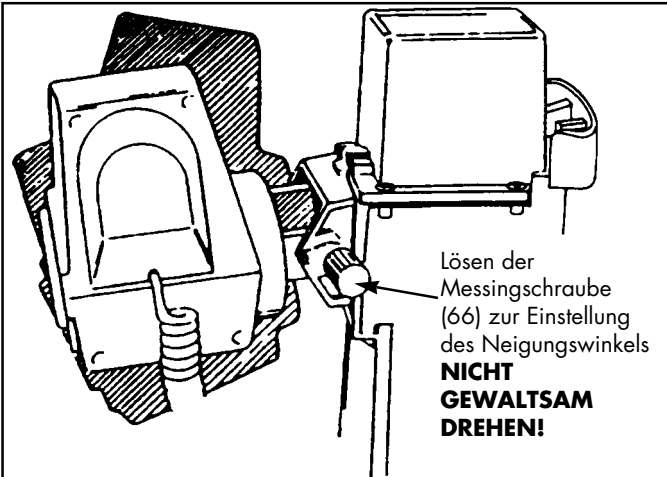
Abbildung 4 EINSTELLUNG DES NEIGUNGSWINKELS
