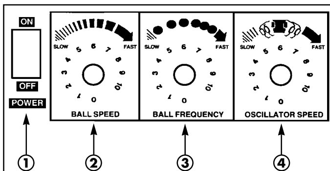
Abbildung 1A Steuergerät für Modell 1040/2040 ANSICHT OBERER TEIL
