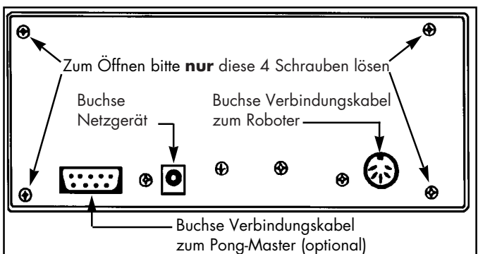
Abbildung 1B Steuergerät für Modell 1040/2040 ANSICHT UNTERER TEIL
