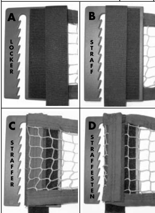
Abbildung 21 JUSTIERUNG DER SEITENNETZ-SPANNUNG (NUR 2040)
