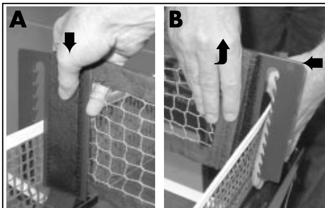
Abbildung 20 MONTAGE UND DEMONTAGE DES SEITENNETZES (NUR 2040)
